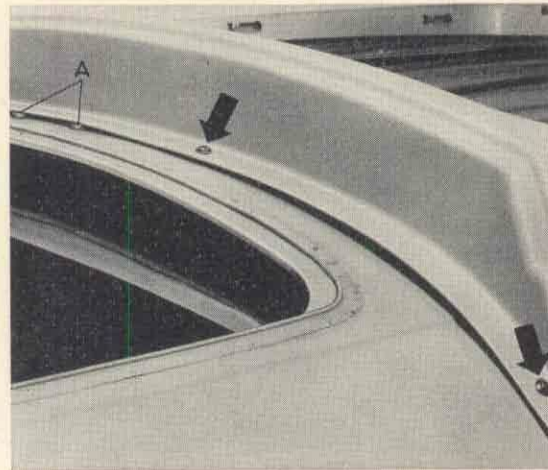
A = Gummi-Unterlegscheiben zwischen den beiden mittleren Kreuzschlitzschrauben
